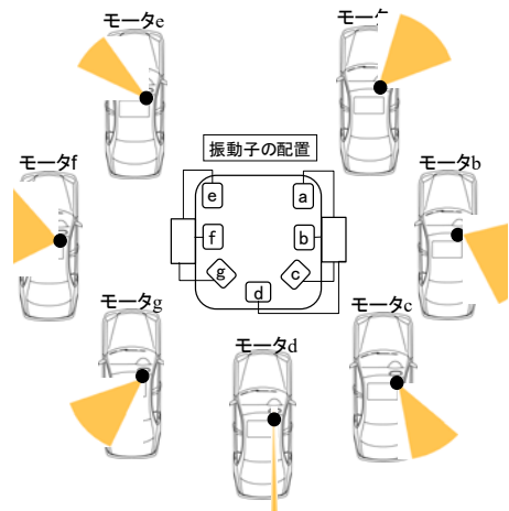
図 2 振動による障害物の方向検知の精度
