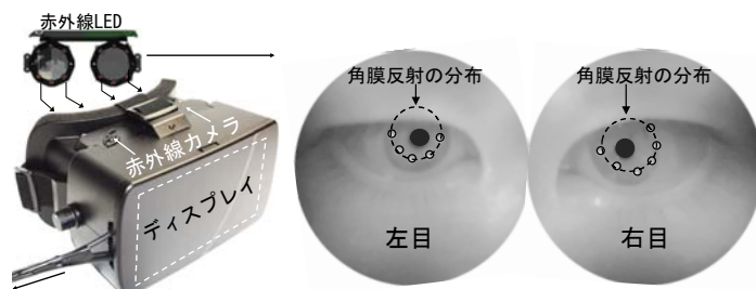
図2 試作した視野検査機器と得られた瞳孔・角膜反射映像
